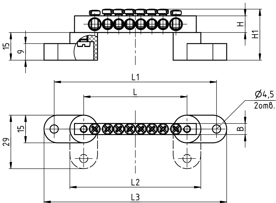
Шина РЕ, N на двух угловых изоляторах
